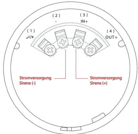
Anschluss Sirene
