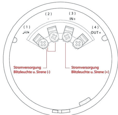
Anschluss Blitzleuchte und Sirene
