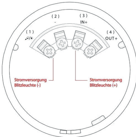
Anschluss Blitzleuchte
